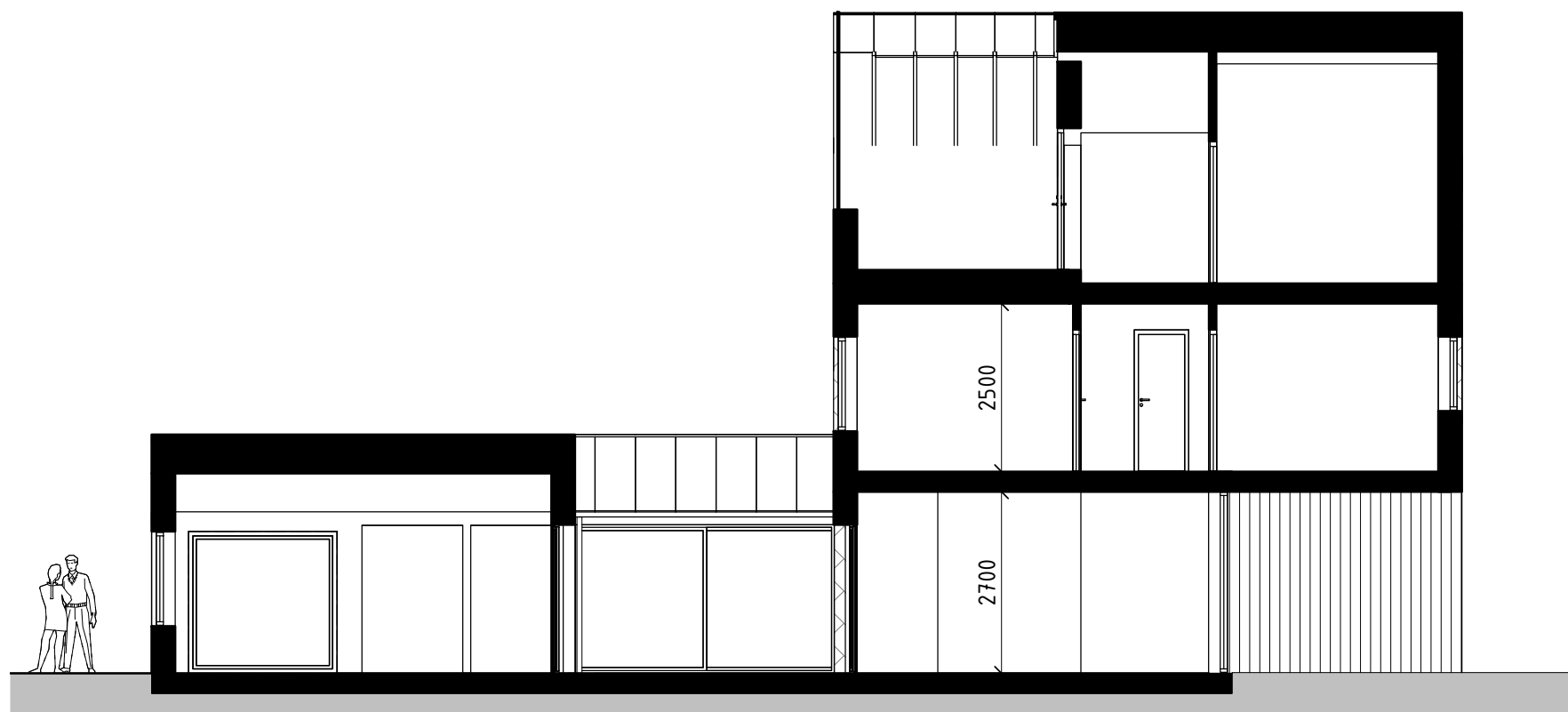
Sektion A-A
