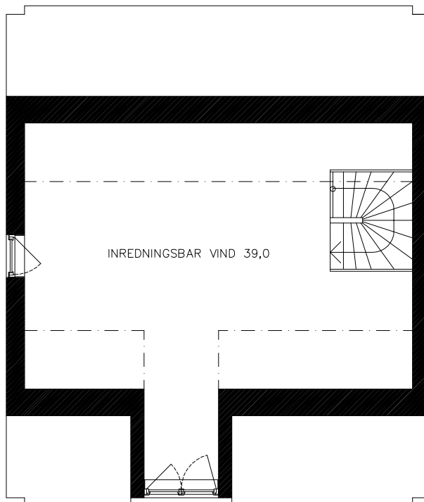
PLAN 3 Vissa tomter kräver spegelvänd planlösning
