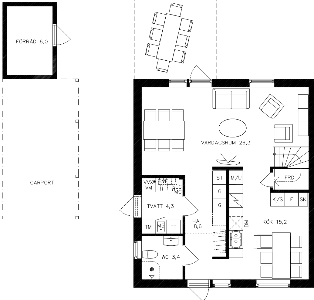
PLAN 1 - Hus A Boyta 61,3 kvm
