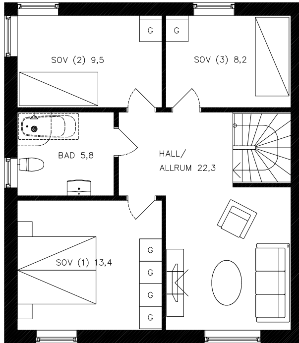
PLAN 2 - Typ 201 (Basutförande) Boyta 61,3 kvm
